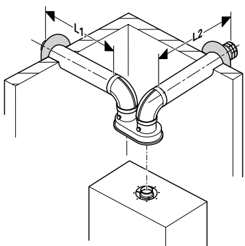
Sistema sdoppiato 2x Ø 80 mm (installazione di tipo C52)
